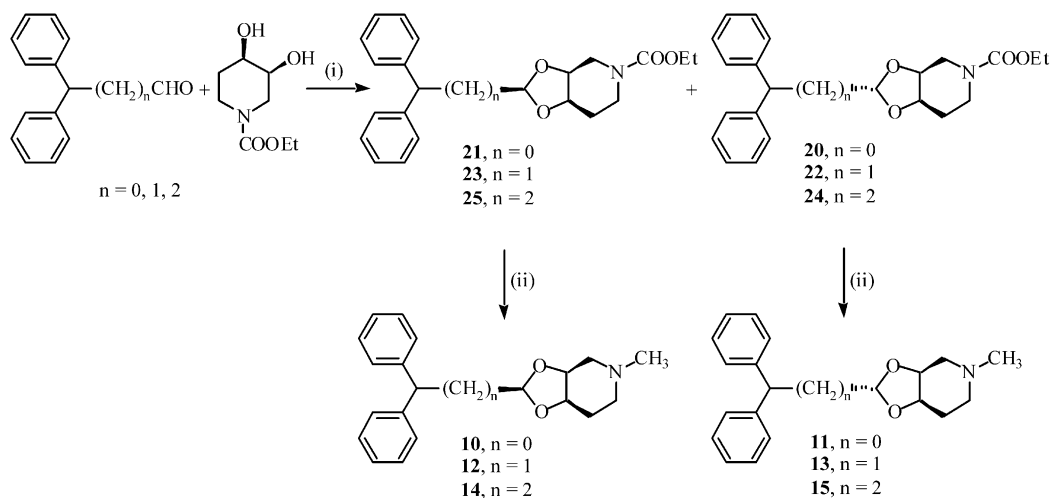
Scheme 3. (i) TsOH, (ii) LiAlH 4 .
